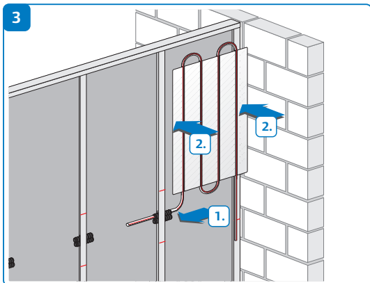
Voor het vastplakken, de aansluitleiding door de mantelbuis in het bouwprofiel invoeren
