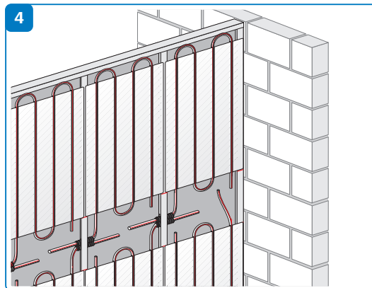
Elementen door persen van de aansluitleidingen met behulp van de Uponor perskoppelingen onderling verbinden
