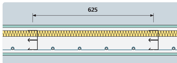
Uponor Siccus SW in dubbele staanderwand
