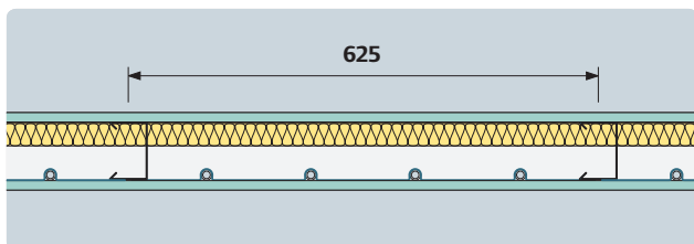
Uponor Siccus SW in enkelvoudige staanderwand
