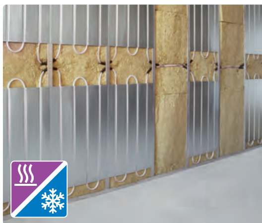
Gedeelte van een staanderwand
