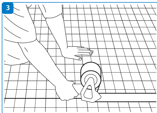
3 Naden tussen de platen goed afplakken met Uponor plakband.
