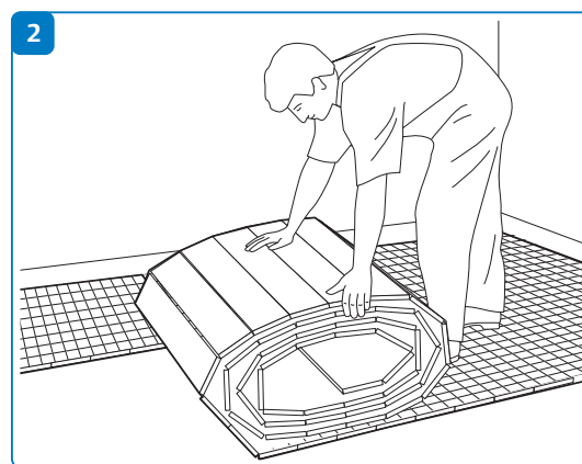
2 Uponor rol- of vouwplaat op een bezemschone ondergrond of extra isolatie leggen.
