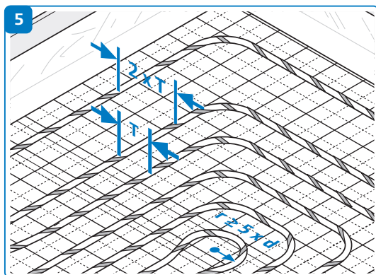
5 Uponor klittenbandleidingen in de berekende afstand op de klittenbandplaten drukken, daarbij de minimale buigradius in acht nemen.
