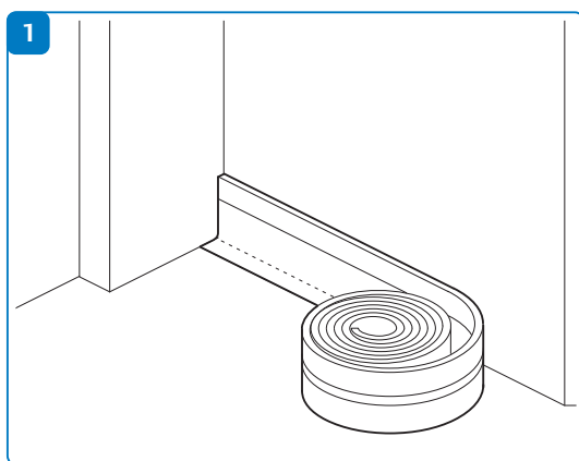
1 Uponor randisolatiestroken met plakstrips tegen alle opstaande bouwdeelen neerzetten.
