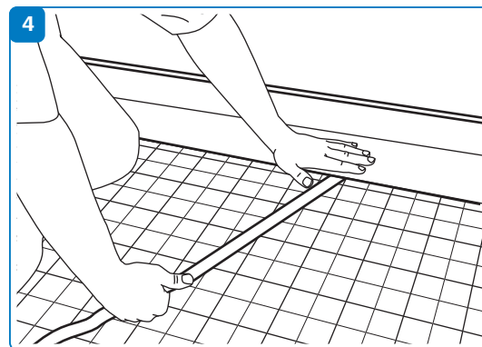
4 De folie van de Uponor randisolatiestroken verwijderen en deze strak op de platen plakken.
