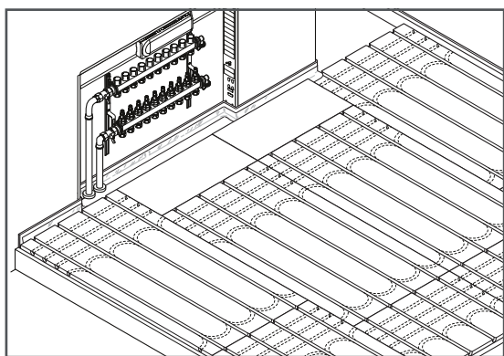
1. Installeer Siccus-panelen
