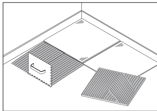
4. Directe betegeling volgens de specificatie
