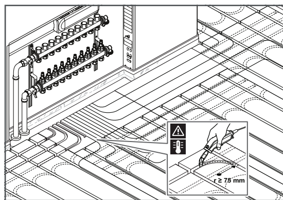
2. Ontbrekende groeven snijden
