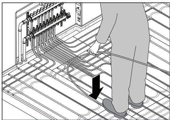
3. Installeer de Uponor verwarmingsleidingen
