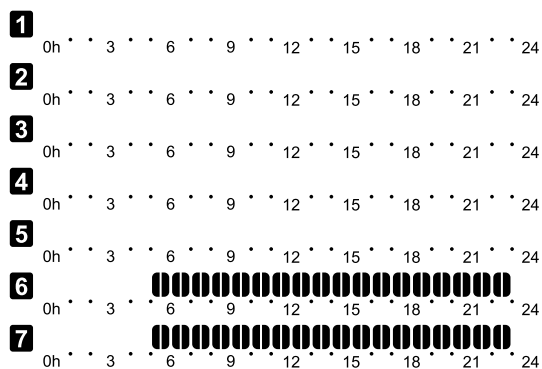
Afbeelding 8. Programma P6
