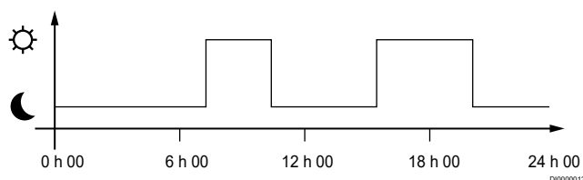
Afbeelding 1. Programma 1
