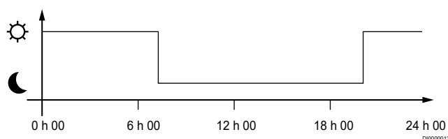
Afbeelding 2. Programma 2
