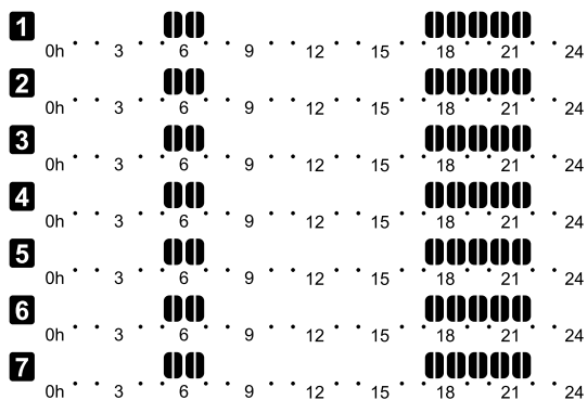
Afbeelding 4. Programma P2
