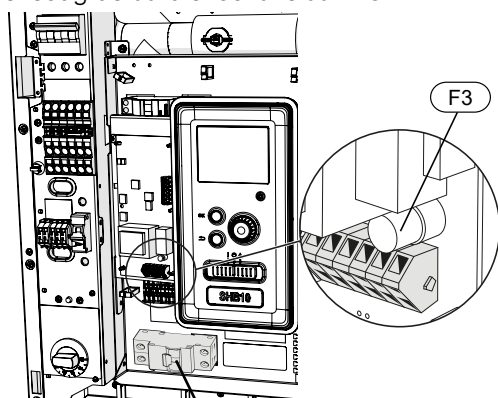
Aardlekschakelaar RCD
