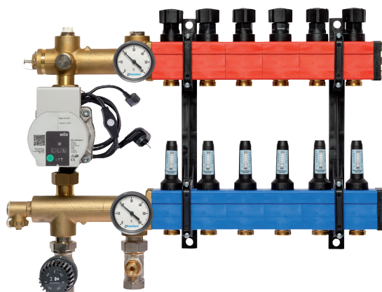
Komfort 4800 25 - 135 l/h
