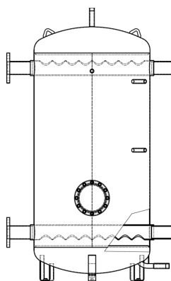
Buffervat cascade
