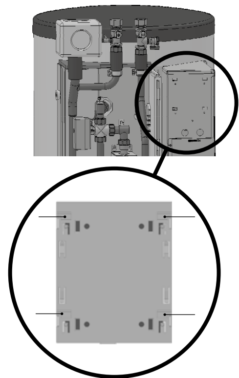
Vier uitsparingen in de schakelkastplaat
